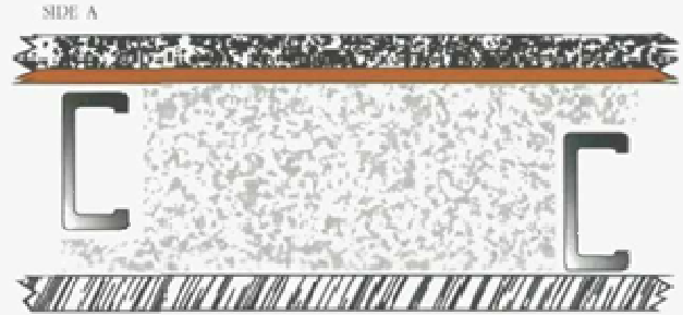
METAL STUD
